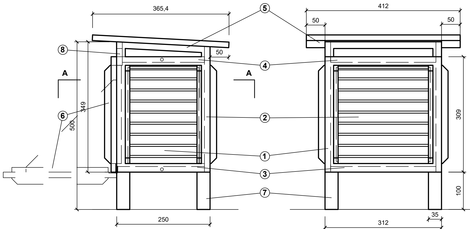
VIEW V1
